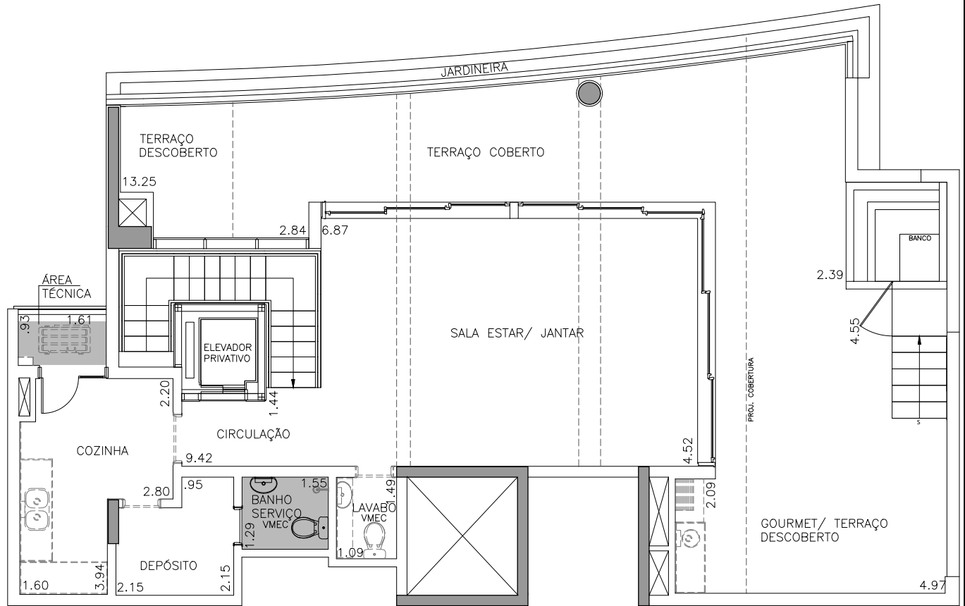
PLANTA - TORRE 2 DUPLEX SUPERIOR - FINAL 4 ÁREA PRIVATIVA DA UNIDADE: 291,02m² SEM ESCALA
