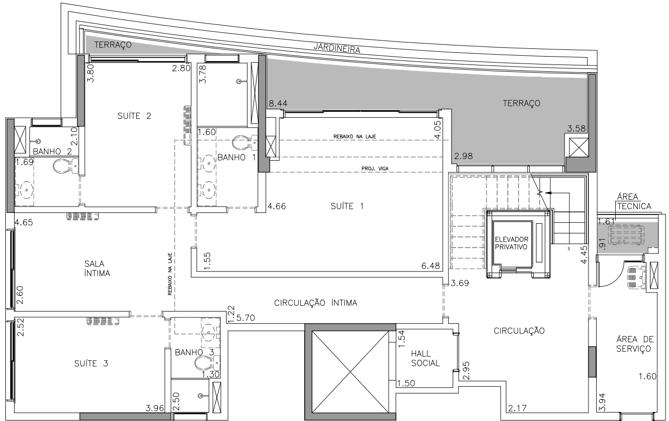
PLANTA - TORRE 2 DUPLEX INFERIOR - FINAL 3 ÁREA PRIVATIVA DA UNIDADE: 291,52m 2 SEM ESCALA
