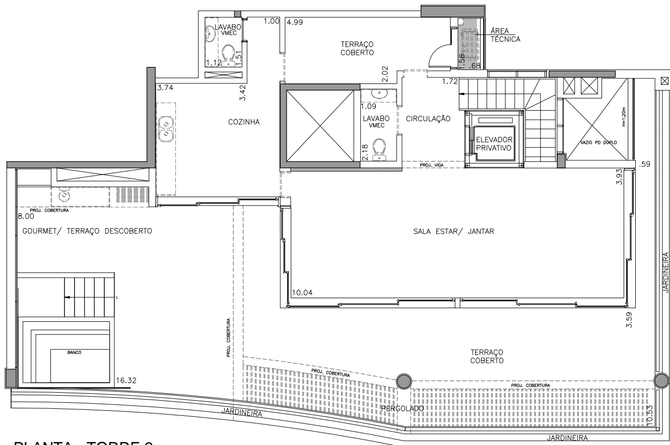
PLANTA - TORRE 2 DUPLEX SUPERIOR - FINAL 2 ÁREA PRIVATIVA DA UNIDADE: 418,98m 2 SEM ESCALA
